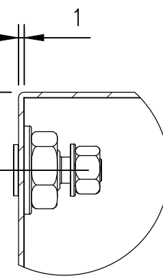
DETAIL A2
