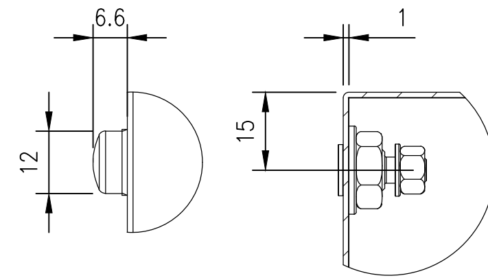
DETAIL A1
