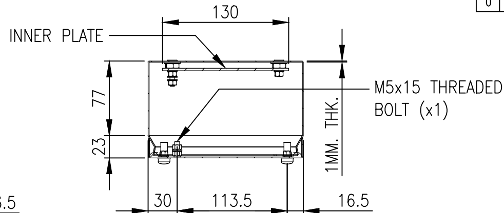
SECTION A-A
