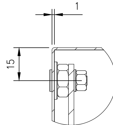
DETAIL A2
