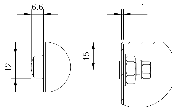
DETAIL A1
